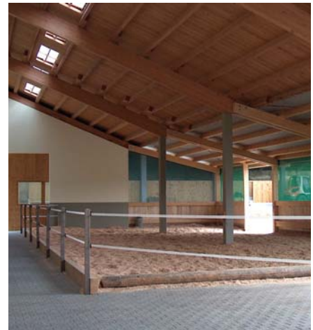
Einer der beiden Offenstallbereiche wurde bereits letzten Winter fertig gestellt (links). Für die zweite Gruppe werden die Erfahrungen des Winters umgesetzt – so wird das Dach weiter herausgezogen, um mehr Wetterschutz zu gewährleisten (rechts).
